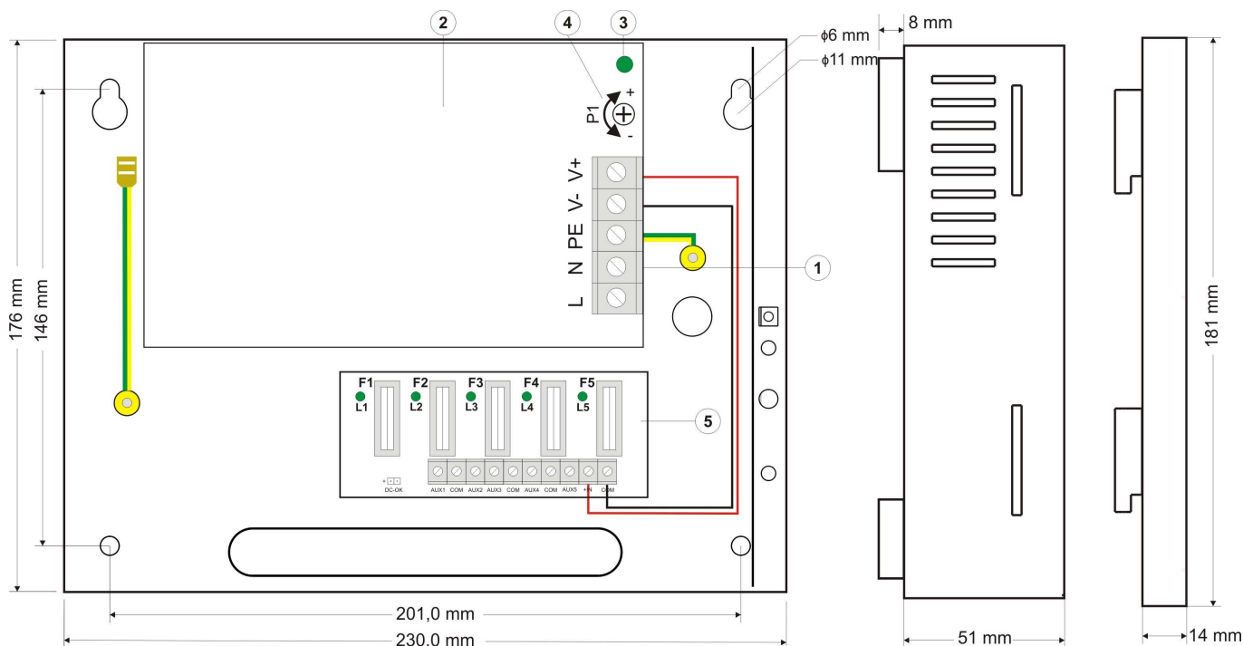
Rys.3. Widok zasilacza.
