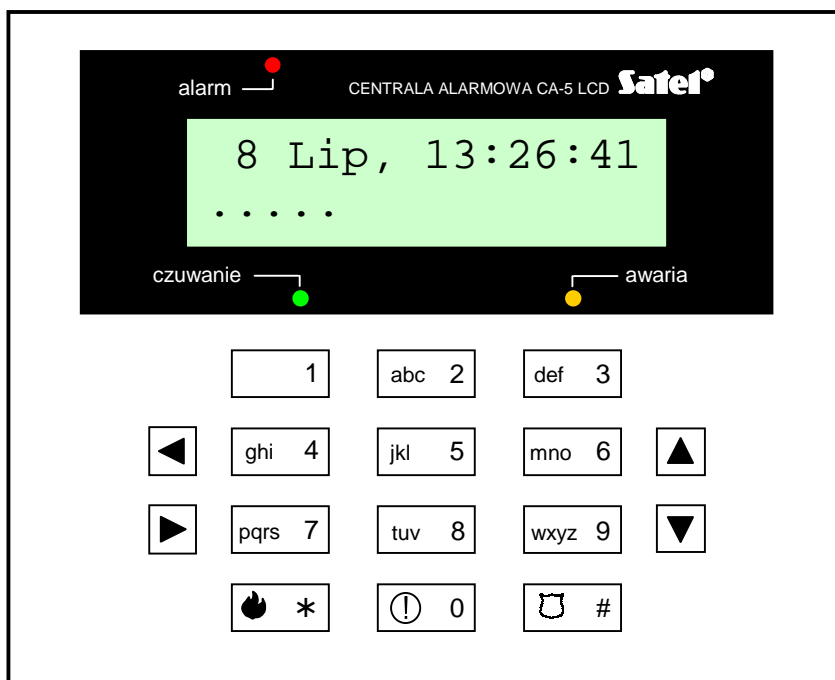
Rysunek 1. Wygląd manipulatora LCD centrali CA-5.
