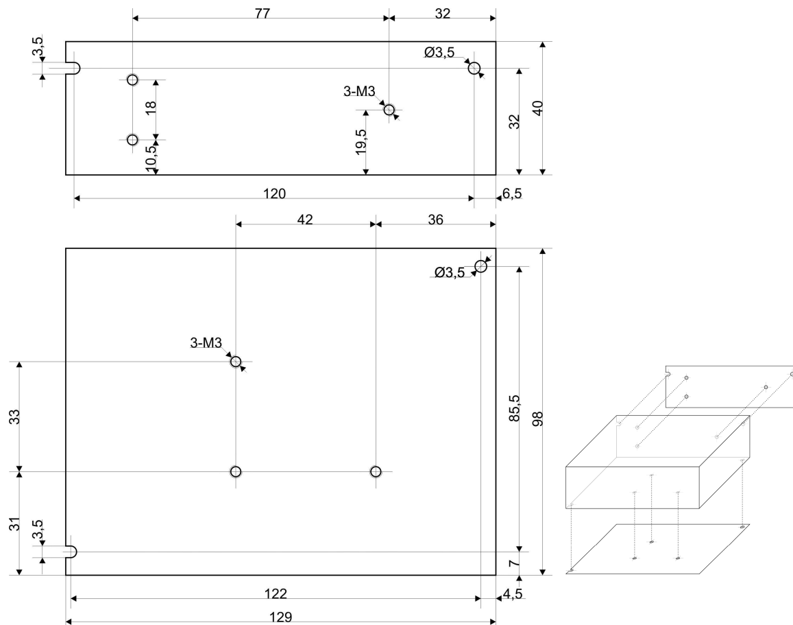
Rys. 1 Rozmieszczenie otworów montażowych dla zasilacza PS401203.
