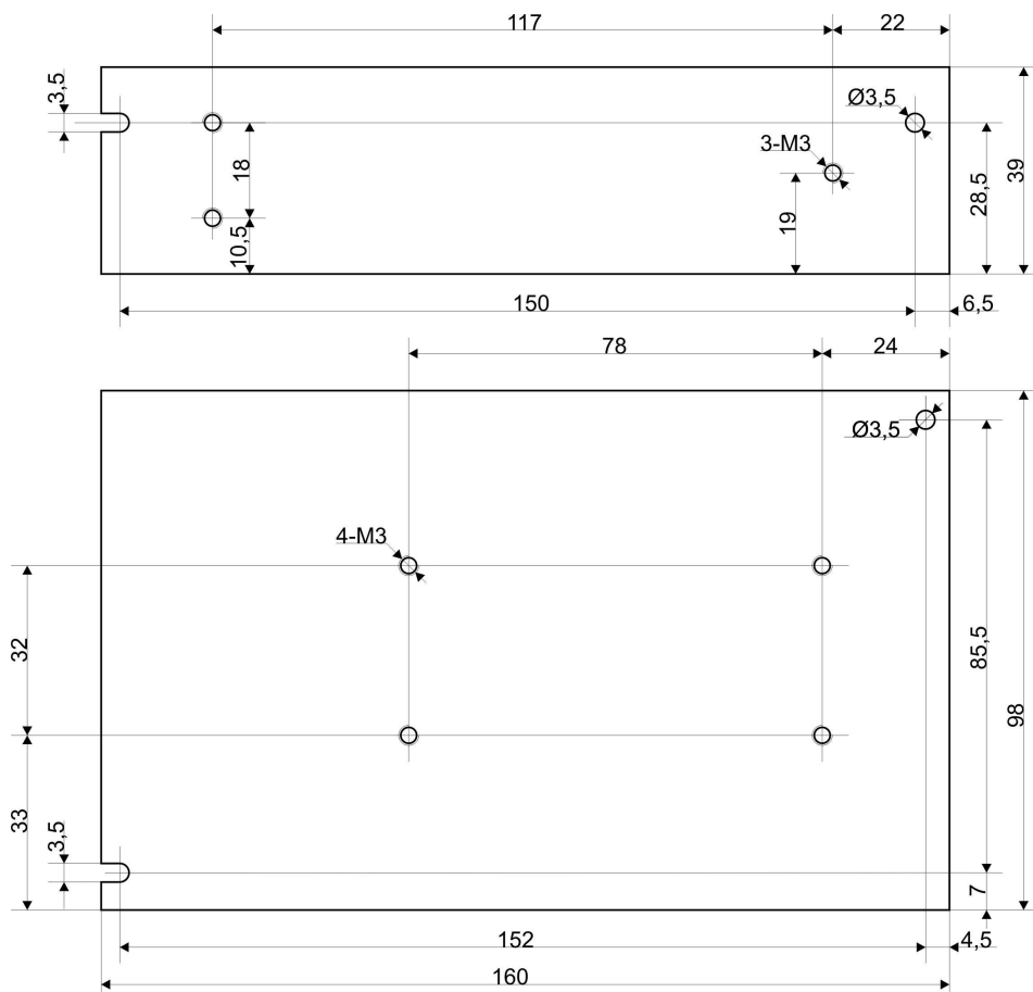
Rys. 2 Rozmieszczenie otworów montażowych dla zasilacza PS701205.
