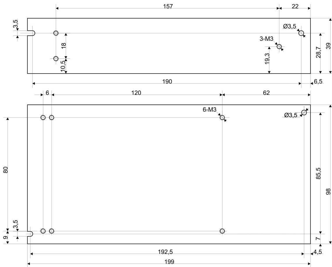
Rys. 3 Rozmieszczenie otworów montażowych dla zasilacza PS1001207.
