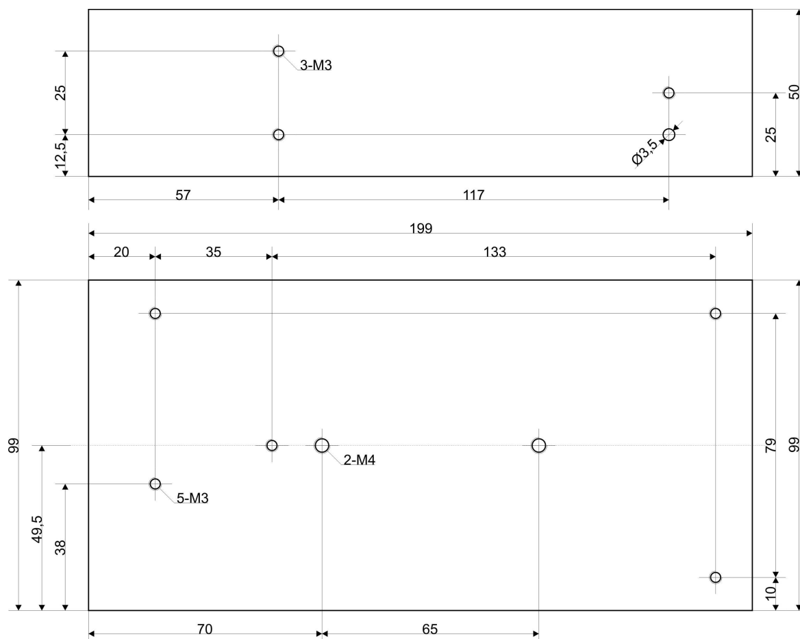
Rys. 4 Rozmieszczenie otworów montażowych dla zasilacza PS1501210.
