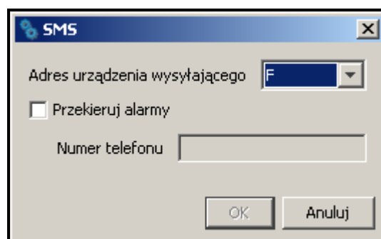
Rys. 27. Okno „SMS”.
