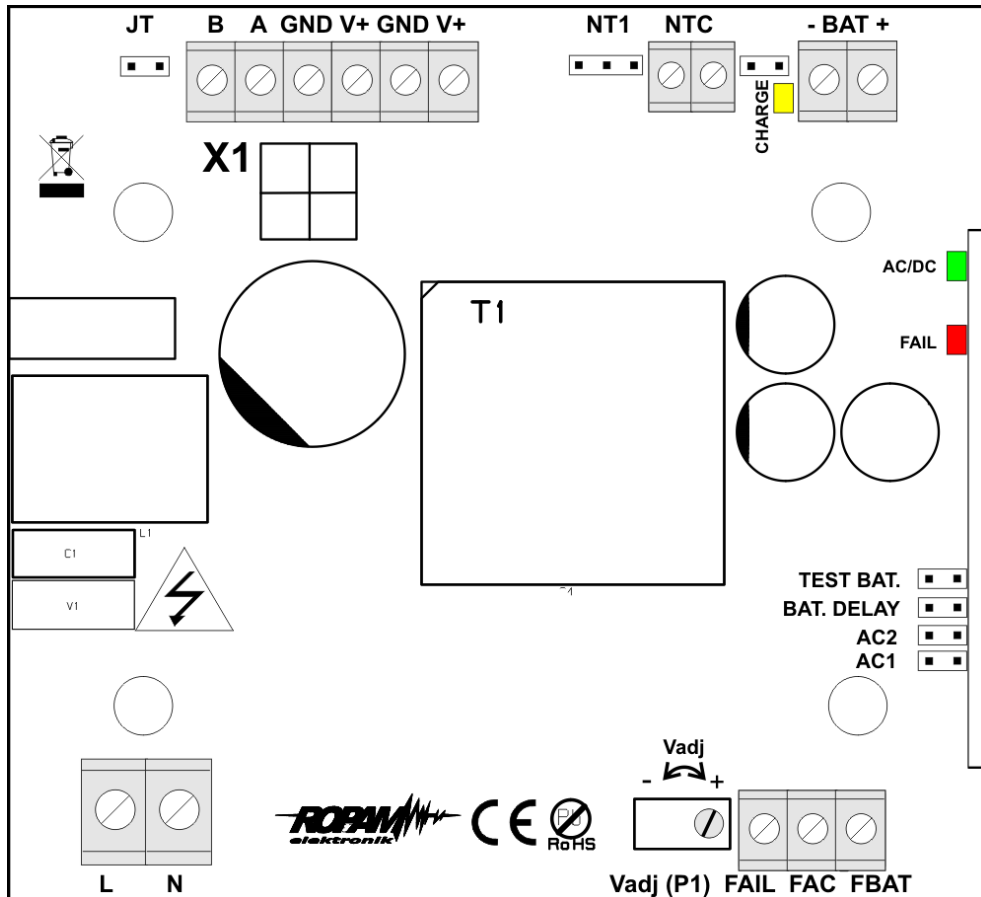
Widok PCB zasilacza PSR-ECO-50120-RN/RS
