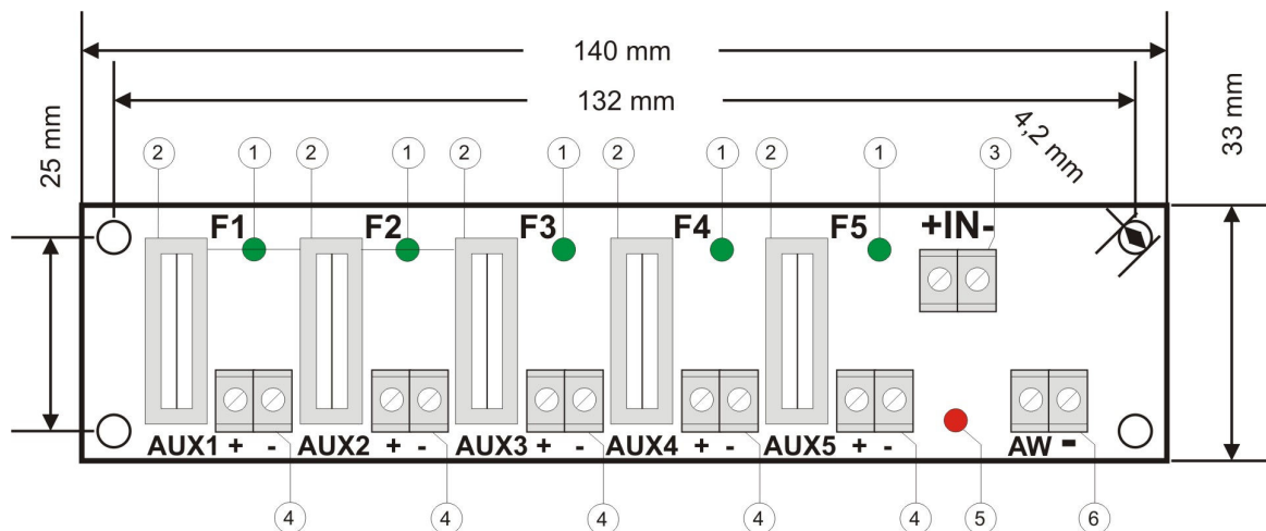
Rys. 4. Widok listwy LB5
