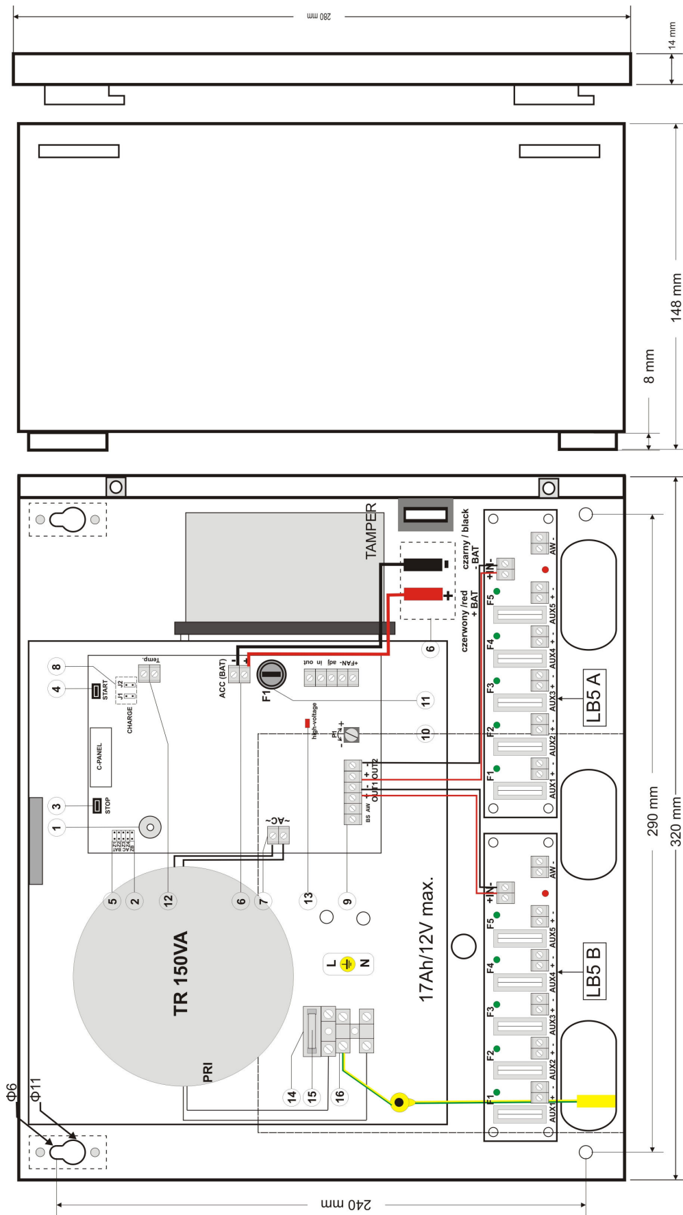
Rys.3 Widok zasilacza. 400 mm
