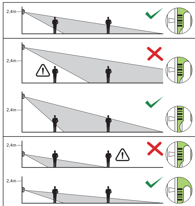
Rysunek 3. Wpływ wysokości montażu na obszar obserwowany przez czujkę i sposób pozycjonowania pyroelementu względem soczewki w celu optymalizacji tego obszaru.
