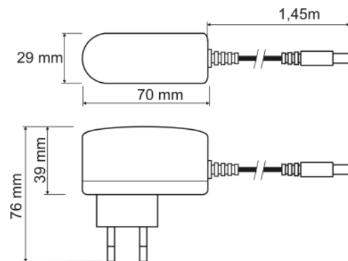
Rys. 1. Widok mechaniczny zasilacza.
