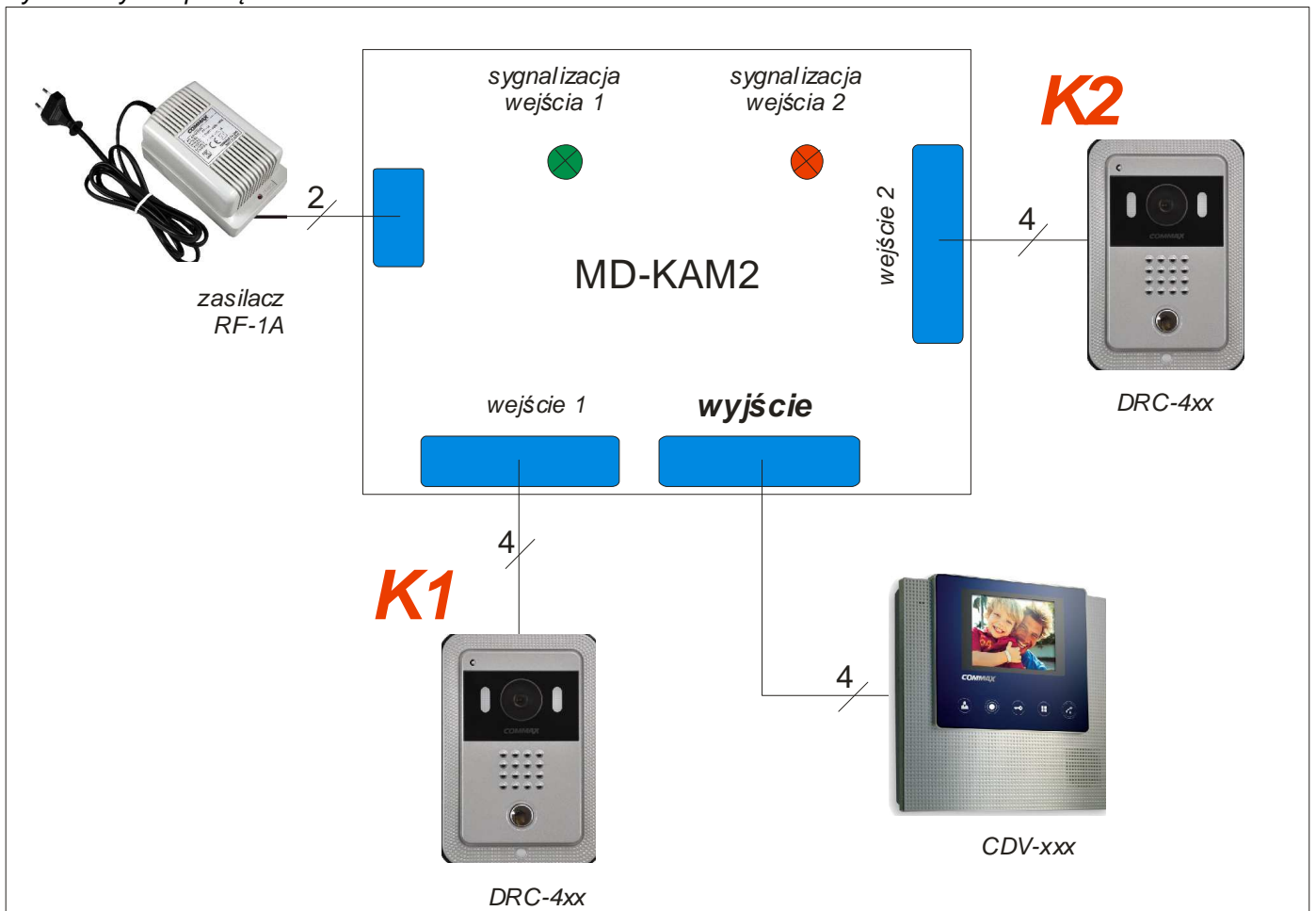
Rys 2. Przykład podłączenia
