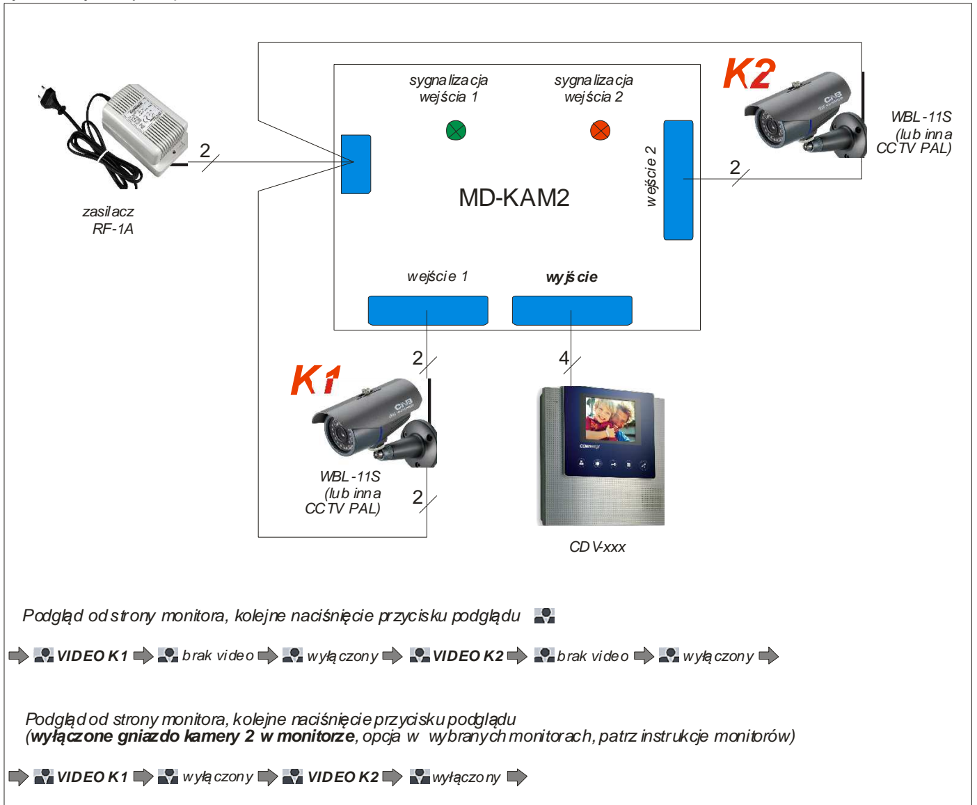
Rys 3. Przykład podłączenia
