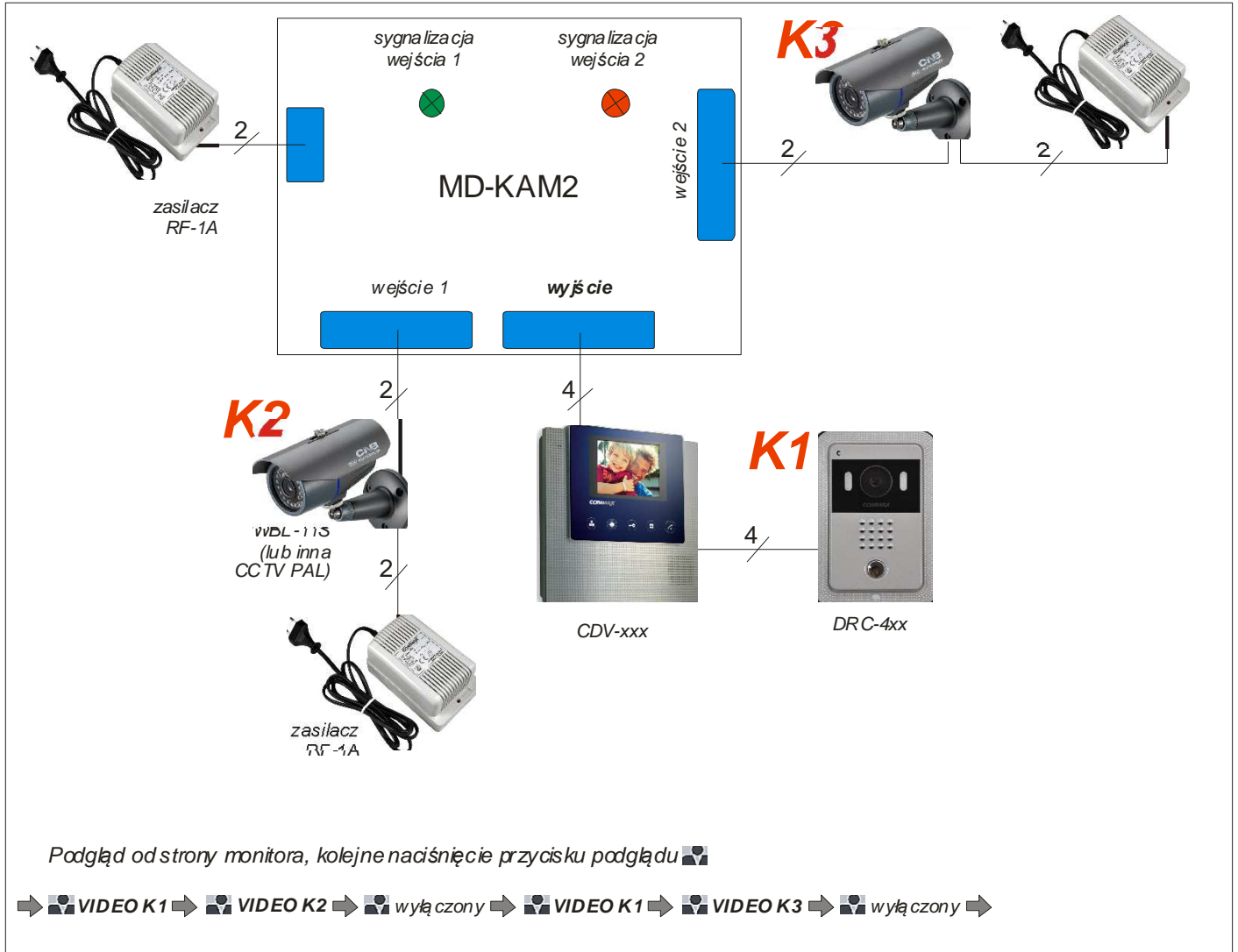
Rys 4 Przykład podłączenia
