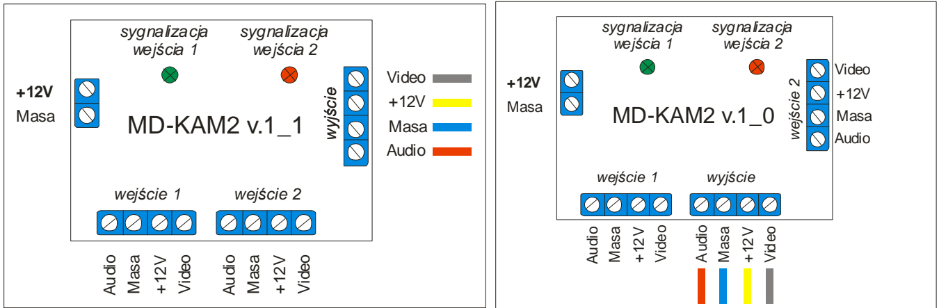
Rys 2. Opis wyprowadzeń (dostępne są 2 wersje różniące się tylko wyprowadzeniami)
