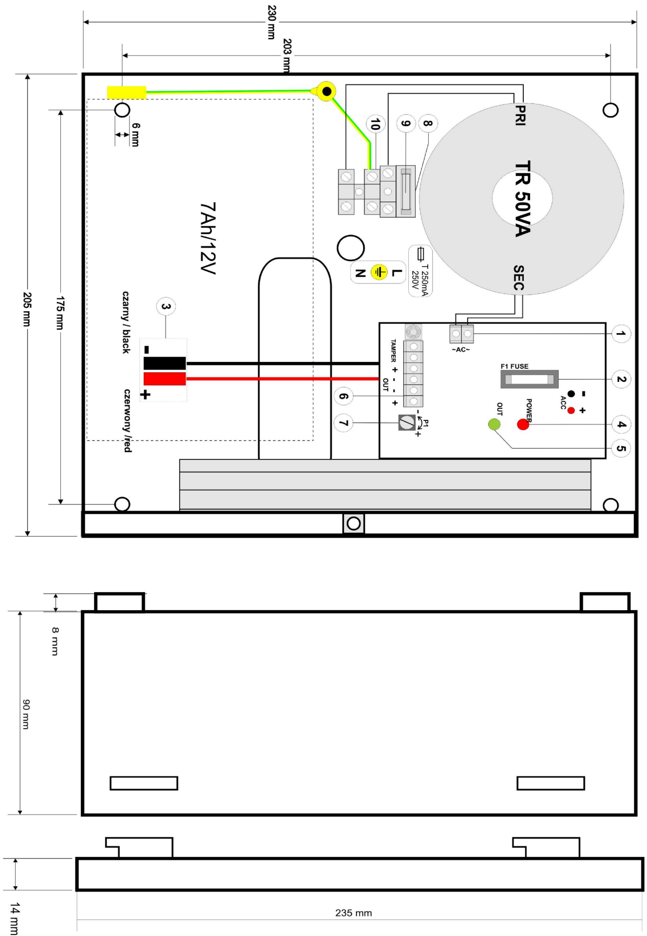
Rys. 3. Widok ogólny zasilacza.
