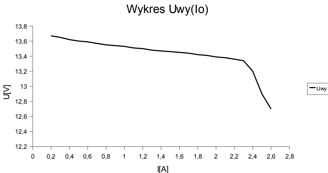
Rys. 2. Charakterystyka prądowo-napięciowa zasilacza.
